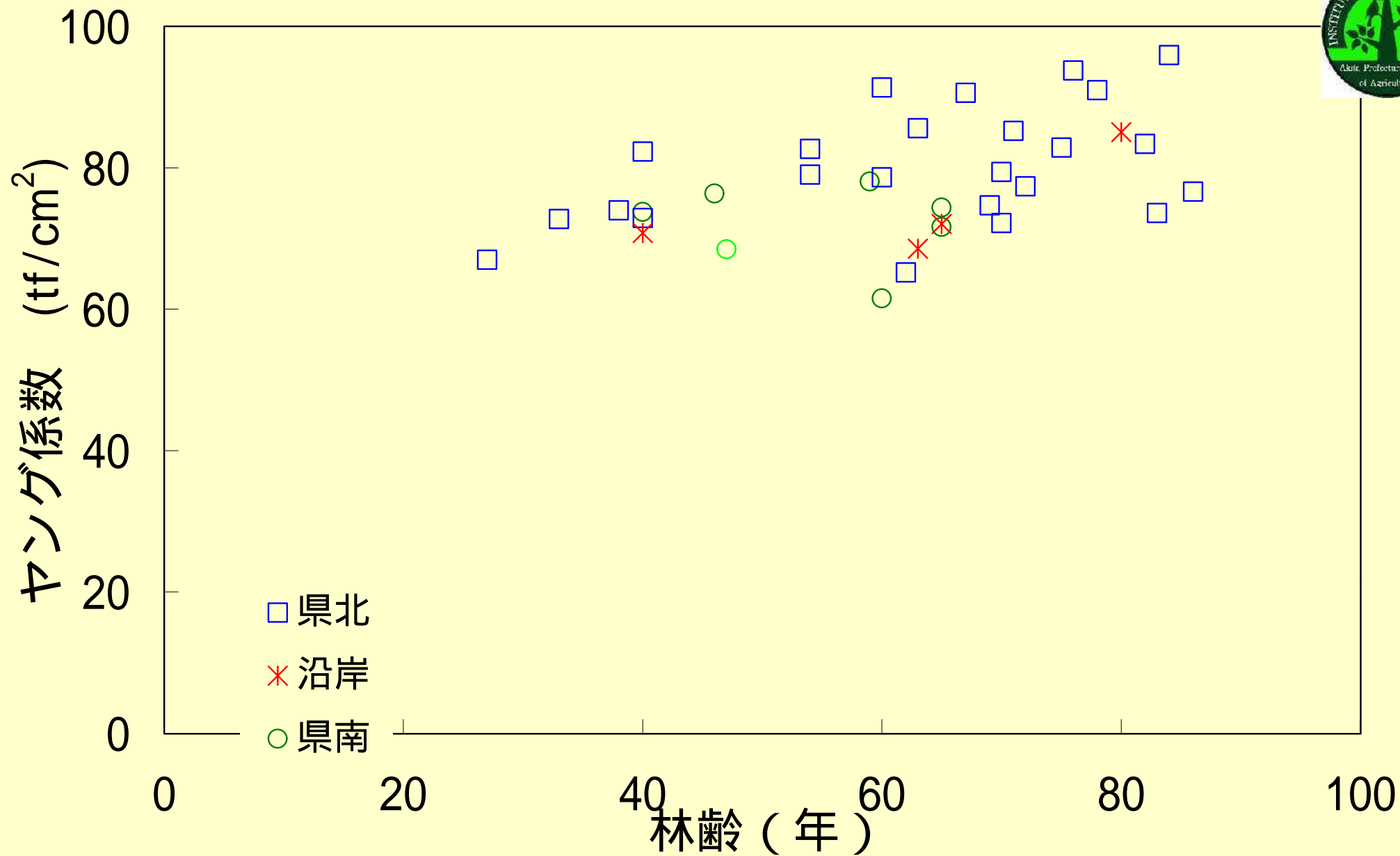
林齢と丸太ヤング係数の関係
